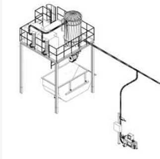
Schema einer Absaugstation mit Zentrale
