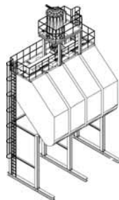
Spänesilo
